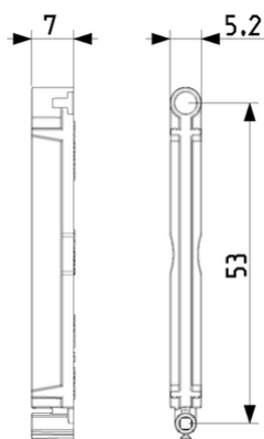
Vista ingombri
