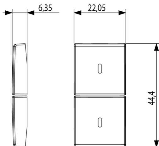
Vista ingombri
