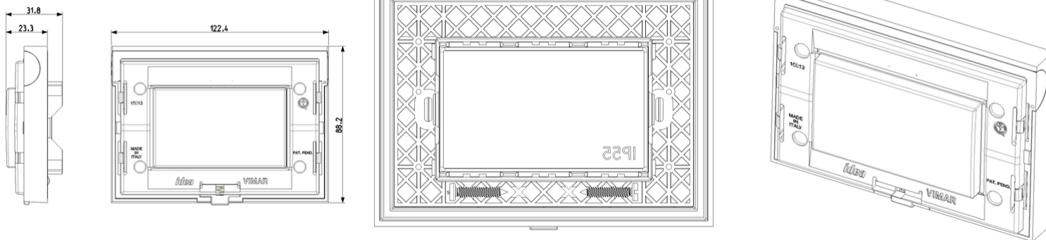
Vista ingombri
