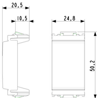
Vista ingombri
