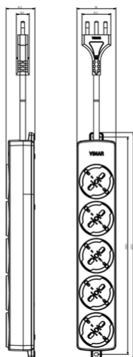
Vista ingombri
