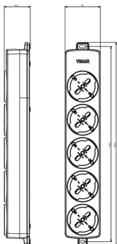
Vista ingombri
