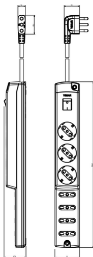
Vista ingombri
