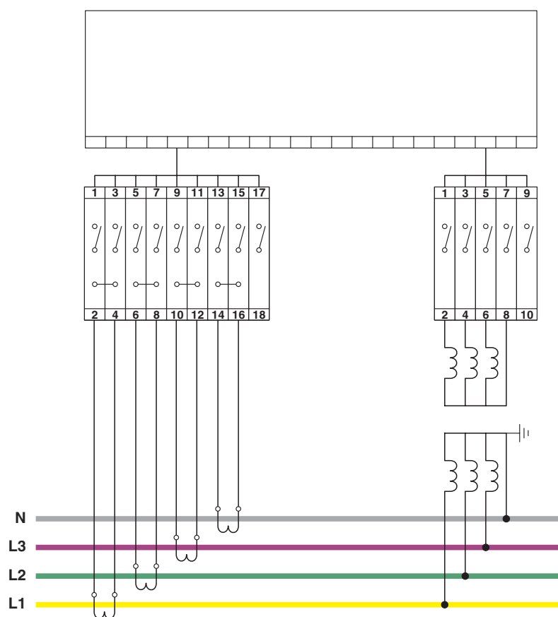
Schema di collegamento
