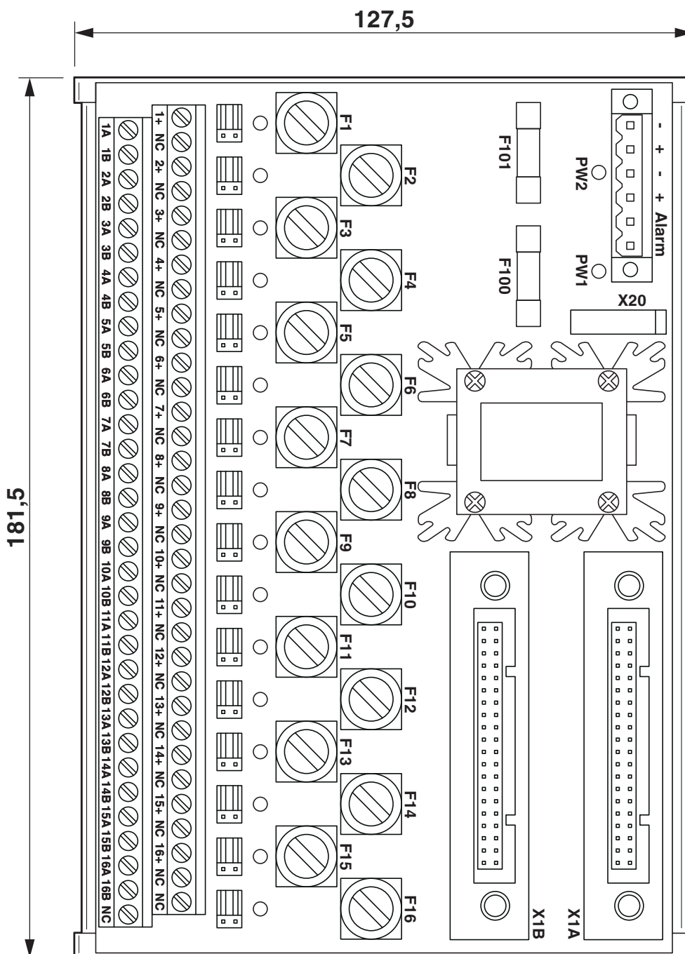
Disegno quotato
