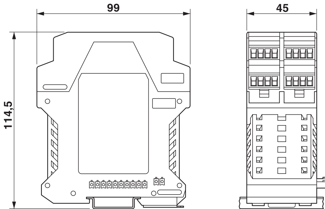
Disegno quotato
