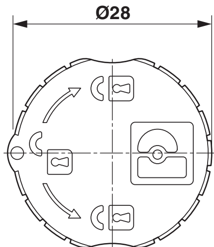
Disegno quotato
