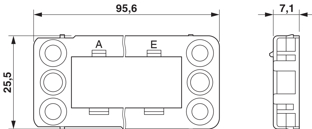
Disegno quotato telaio da incasso
