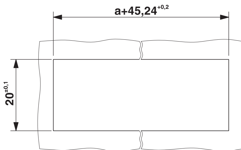
Disegno quotato
