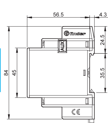
Tipo 8A.26-060x Morsetti a bussola
