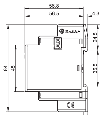
Tipo 8A.58-160x Morsetti a bussola
